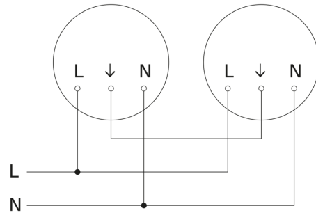
aansluitschema master/master
